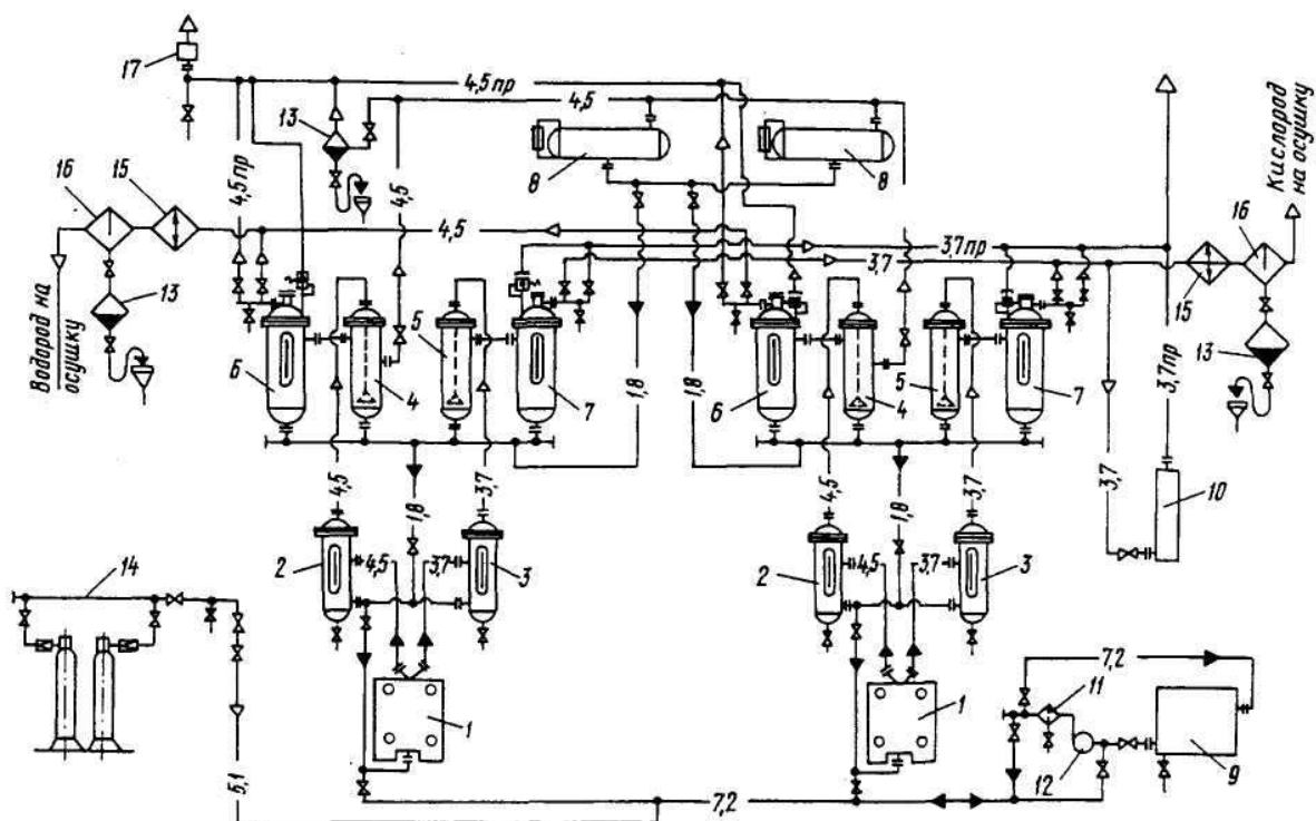
Рис. 3. Технологическая схема ЭУ СЭУ-20×2 с разделительными регуляторами давления и промывателями газов:
