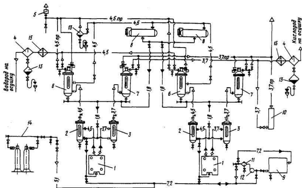
Рис. 4. Технологическая схема ЭУ СЭУ-20×2 с совмещенными регуляторами-промывателями:
