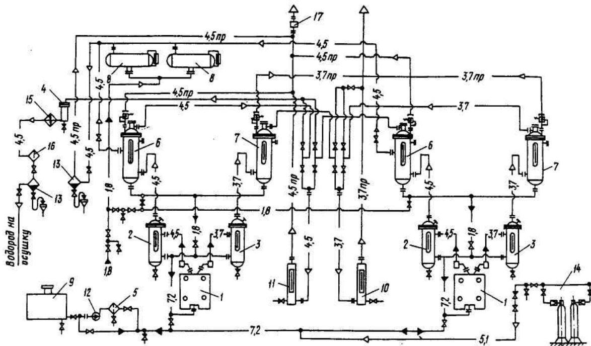
Рис. 2. Технологическая схема ЭУ СЭУ-10М×2:
