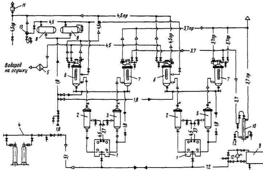
Рис. 1. Технологическая схема ЭУ СЭУ-4М×2:
